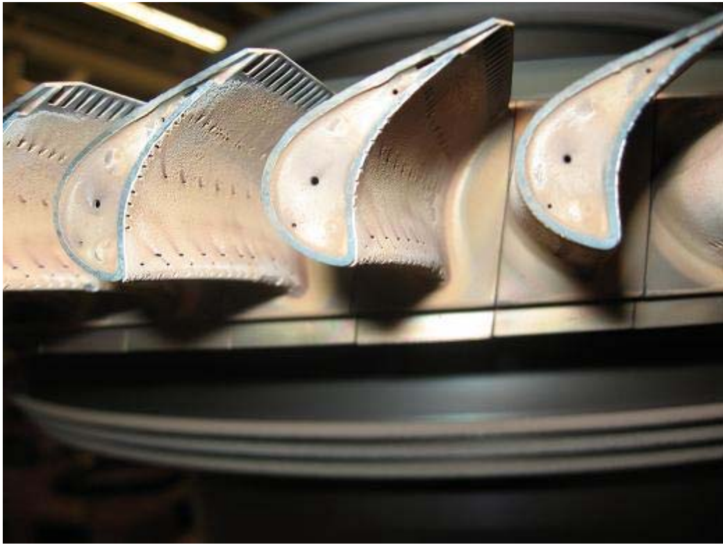
HPT blades
